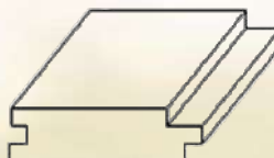
Profil joint-ouvert
