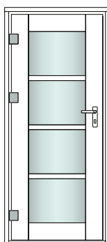
NH-ET-GV1-QS Épaisseur du mur (madrers): 15mm Dimensions (I/L): 84x194cm
