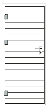
MH-ET-GG-WB Épaisseur du mur (madrers): 15mm Dimensions (I/L): 84x194cm
