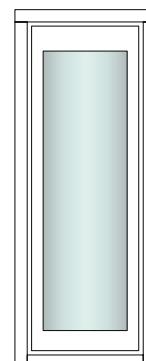
F45-EBF-FEST Épaisseur du mur (madrers): 45mm Dimensions (I/L): 70x191,5cm
