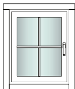
F28-EF Épaisseur du mur (madrers): 28mm Dimensions (I/L): 75x92cm
