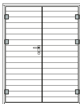
MH-DT-GG-WB Épaisseur du mur (madrers): 15mm Dimensions (I/L): 150x194cm
