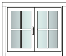
F28-DF Épaisseur du mur (madrers): 28mm Dimensions (I/L): 110x92cm
