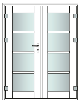
NH-DT-GV1-QS Épaisseur du mur (madrers): 15mm Dimensions (I/L): 150x194cm
