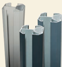
POTEAU GRAND VENT 3 EN 1 Se positionne en début, milieu et fin de clôture. 70 x 64 x 1 260 mm et 70 x 64 x 2 315 mm
