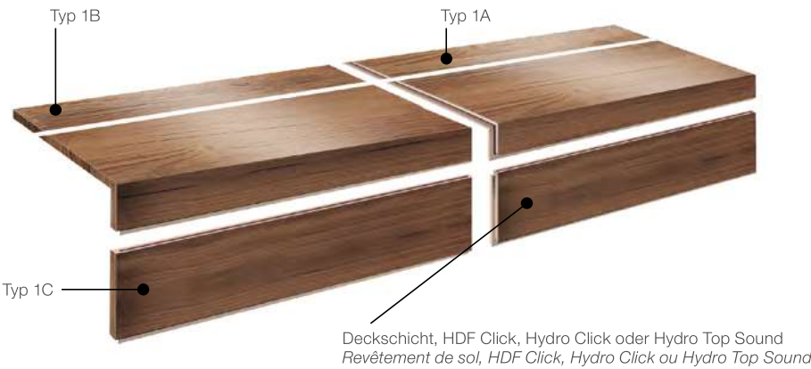
Treppenkante klassisch für einseitig freistehende Treppen Nez de marche classique pour escaliers autoportants d'un côté
