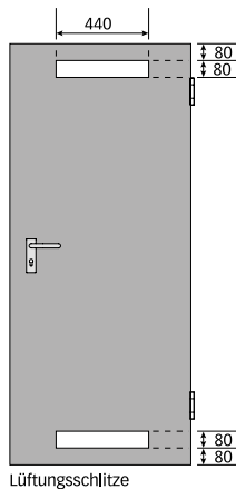
Lüftungsschlitze
