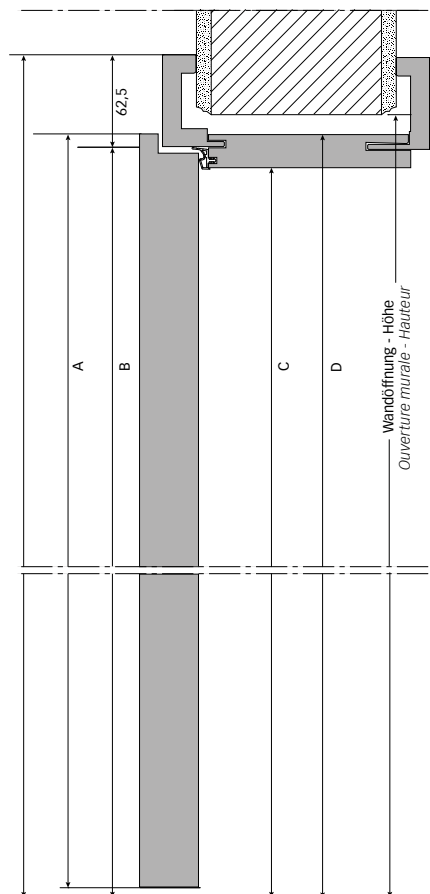
Höhenschnitt gefälzt Section verticale à feuilure
